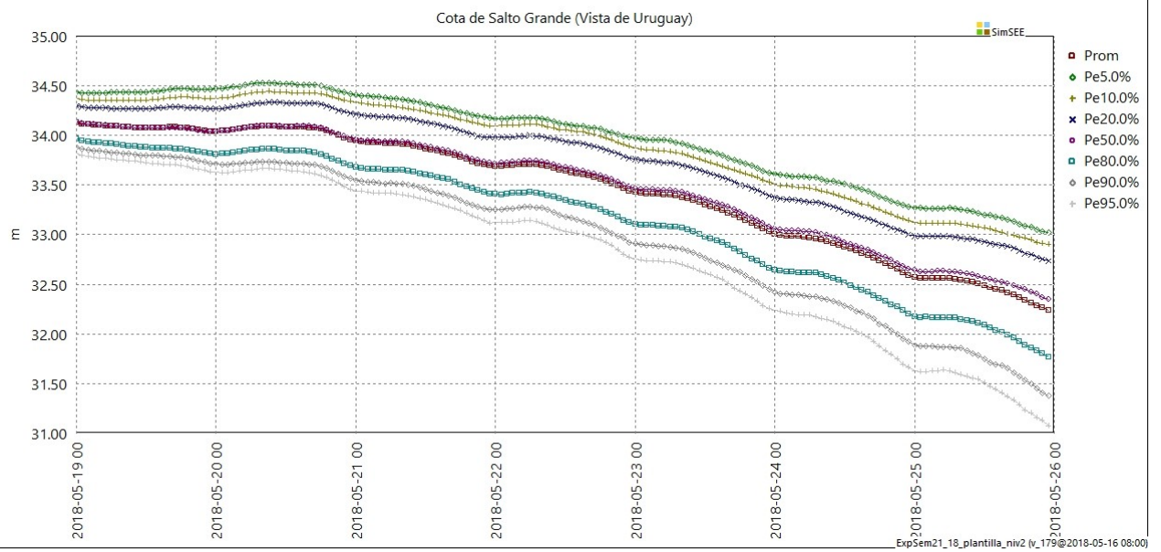
Fig 39: Operación de Salto Grande Uruguay
