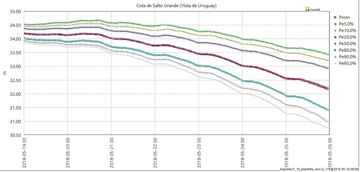
Fig 48: Operación de Salto Grande Uruguay
