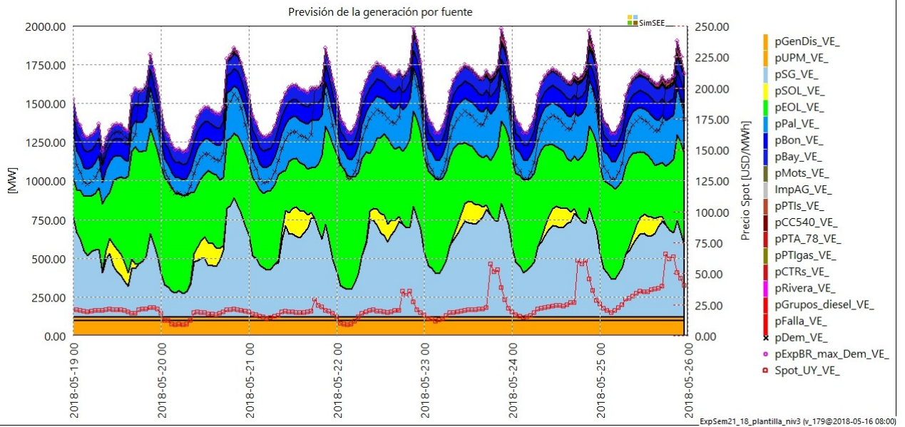
Fig 44: Generación esperada por fuente.
