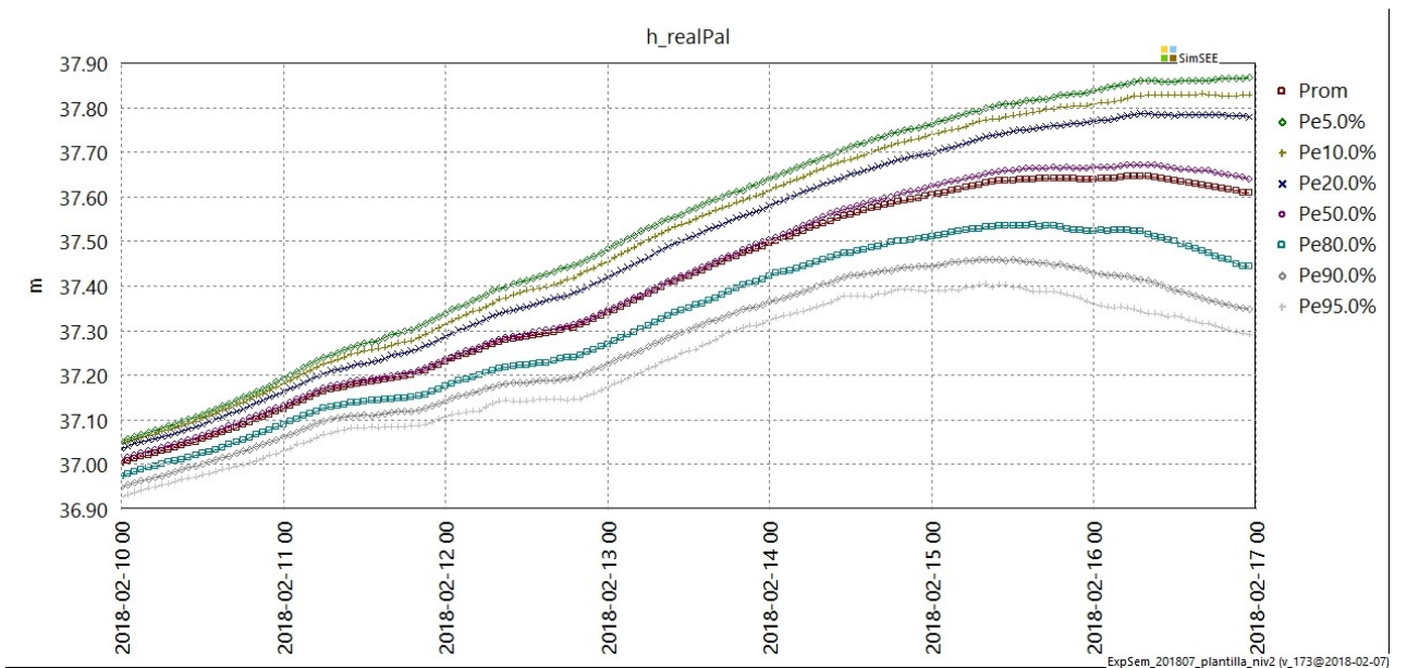
Fig 37: Operación del Palmar.
