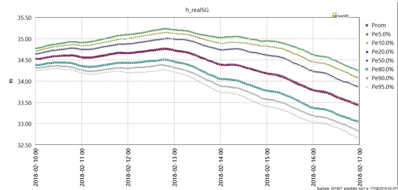
Fig 29: Operación de Salto Grande. (mitad Uruguay).
