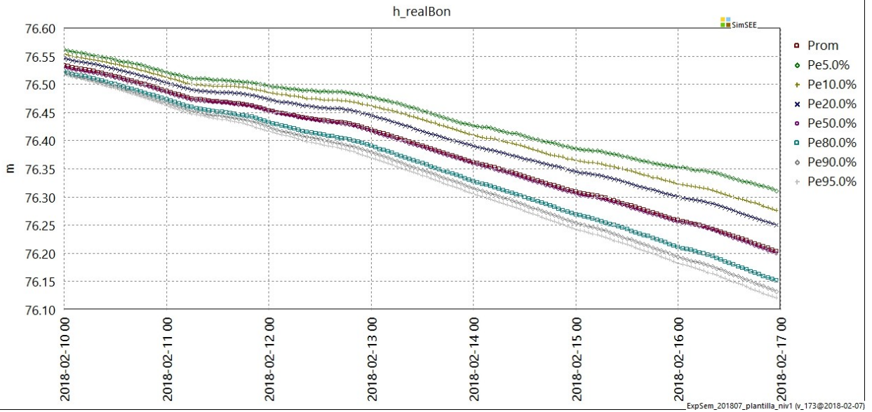
Fig 27: Operación de Bonete
