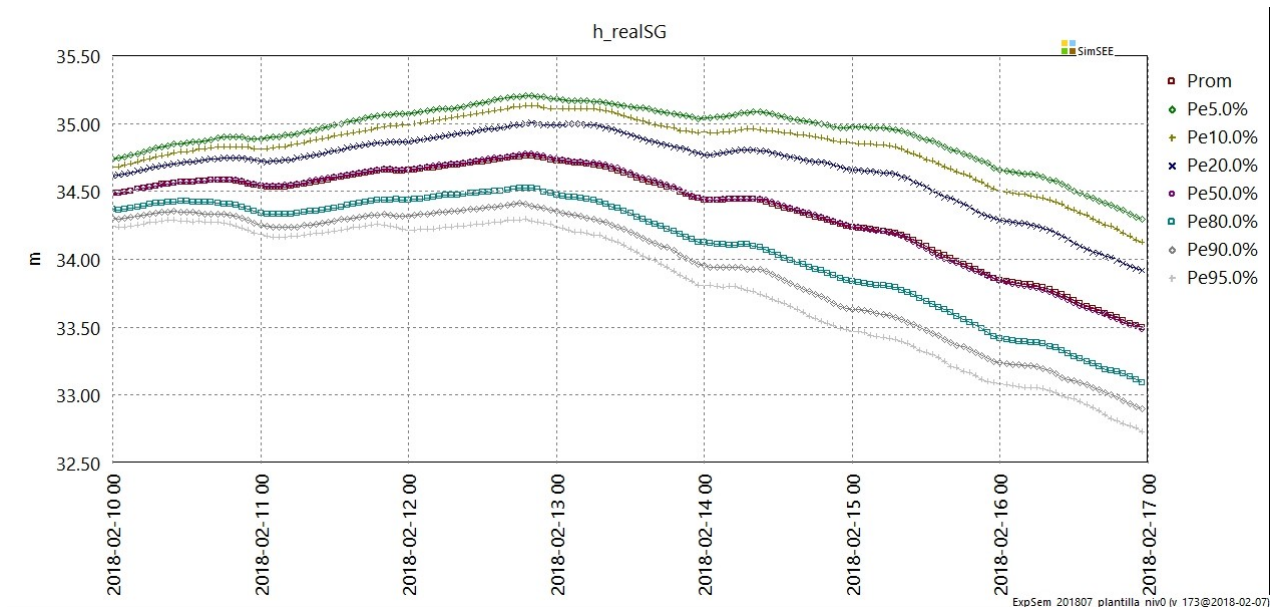
Fig 20: Operación de Salto Grande. (mitad Uruguay).
