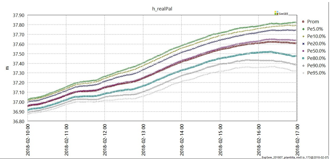
Fig 19: Operación del Palmar.
