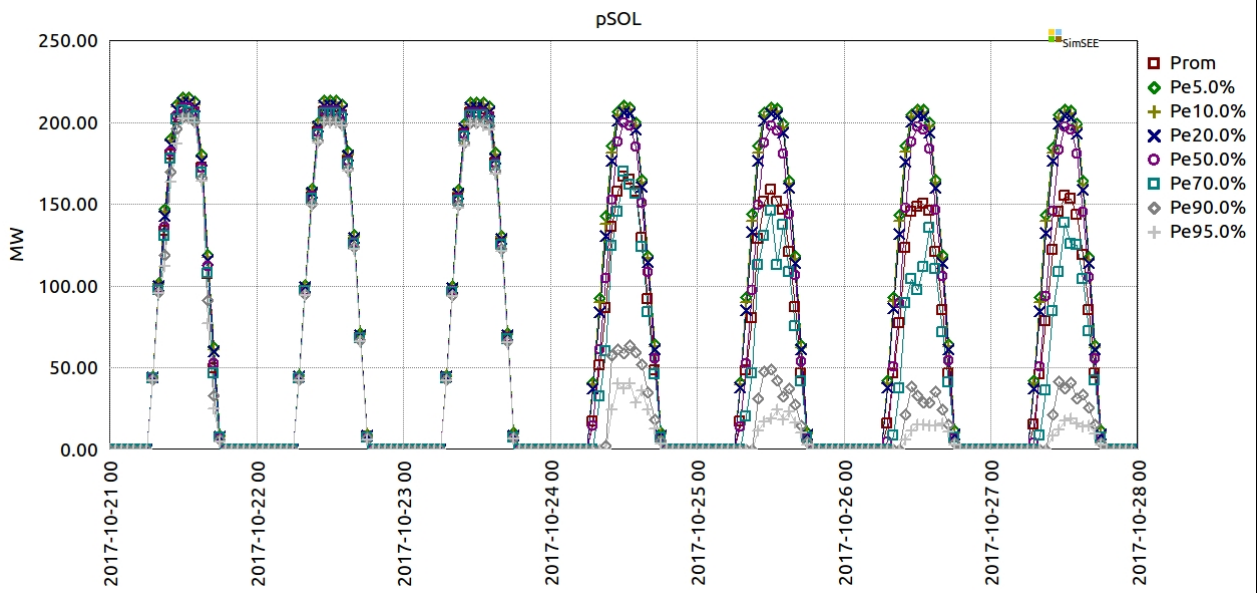
Fig 6: Generación solar.
