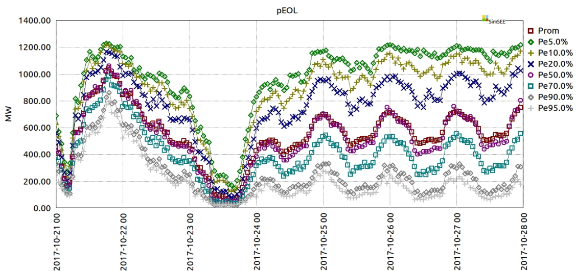
Fig 4: Generación eólica cortes de probabilidad en horas Excluyendo VECODESA.
