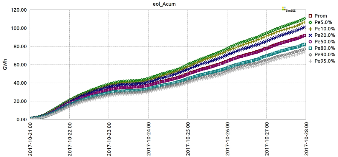
Fig 5: Producción eólica. GWh acumulados desde el inicio de la semana. Excluyendo VECODESA
