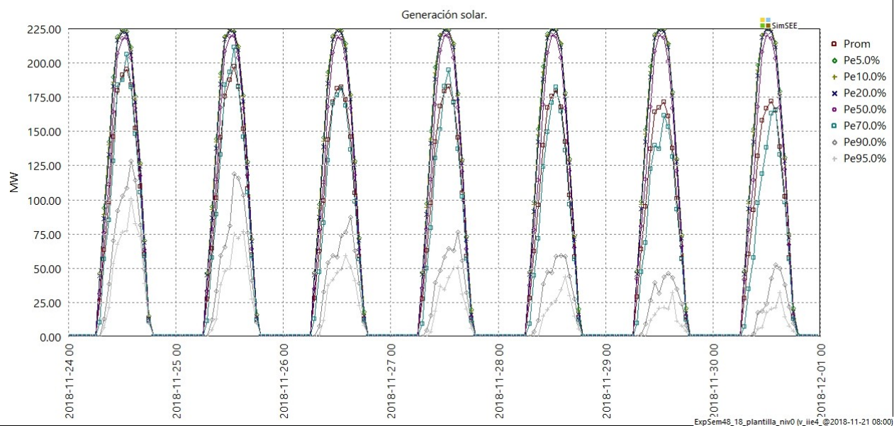
Fig 7: Generación solar.
