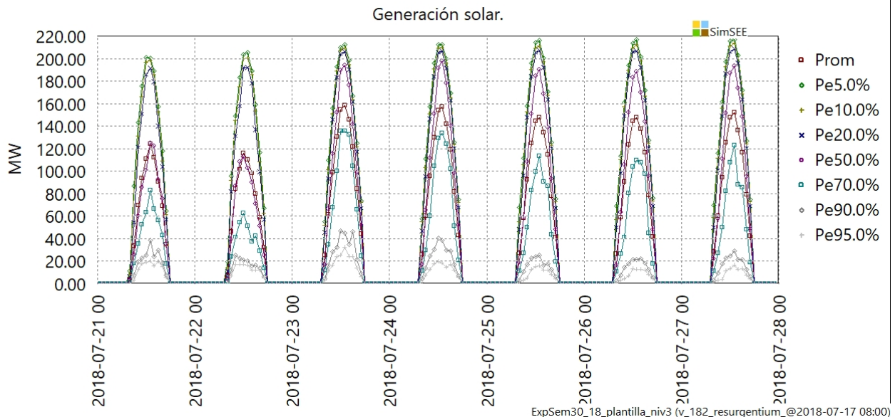
Fig 7: Generación solar.
